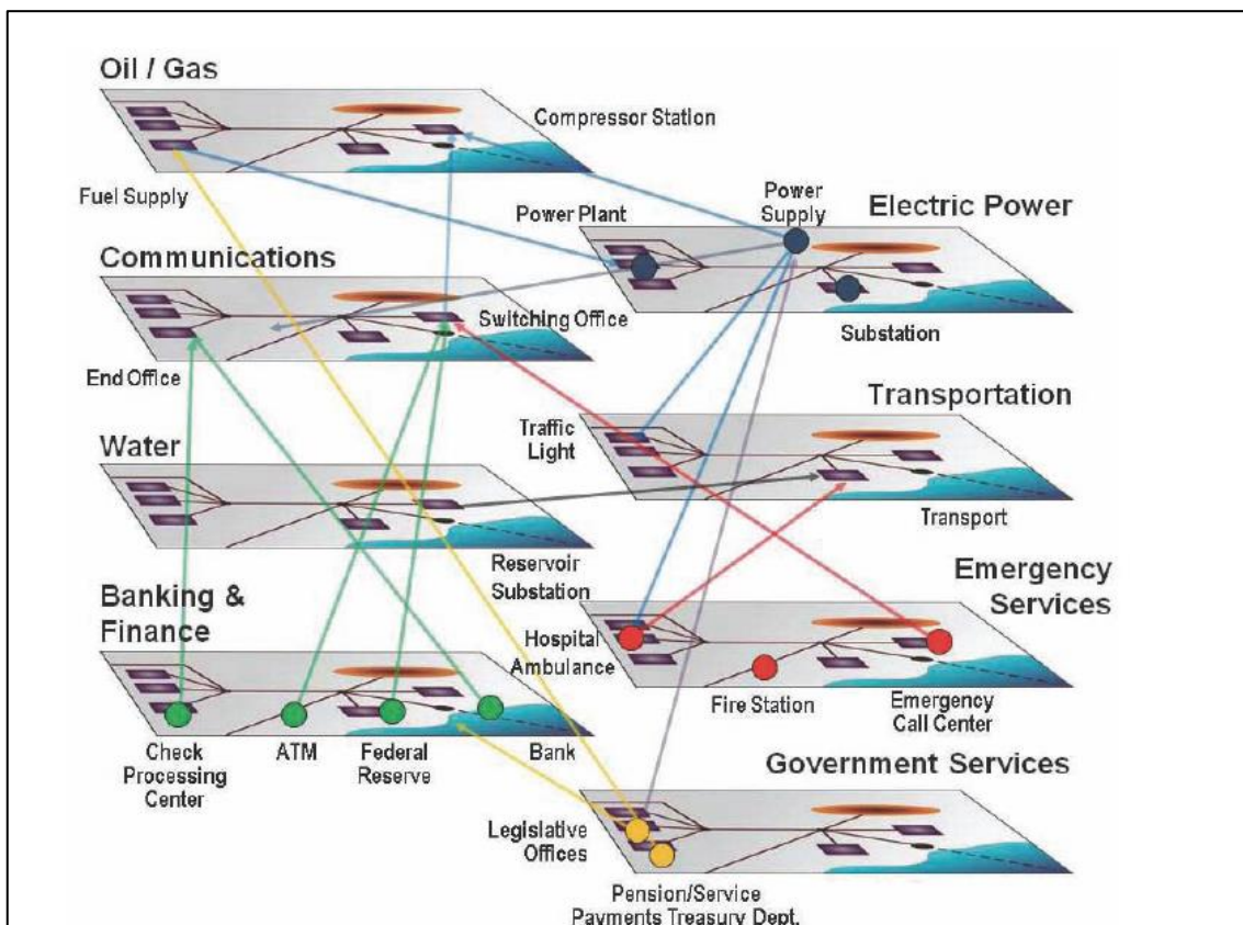
Figura 2. Interconexiones en los elementos de Control de las Infraestructuras Críticas.
